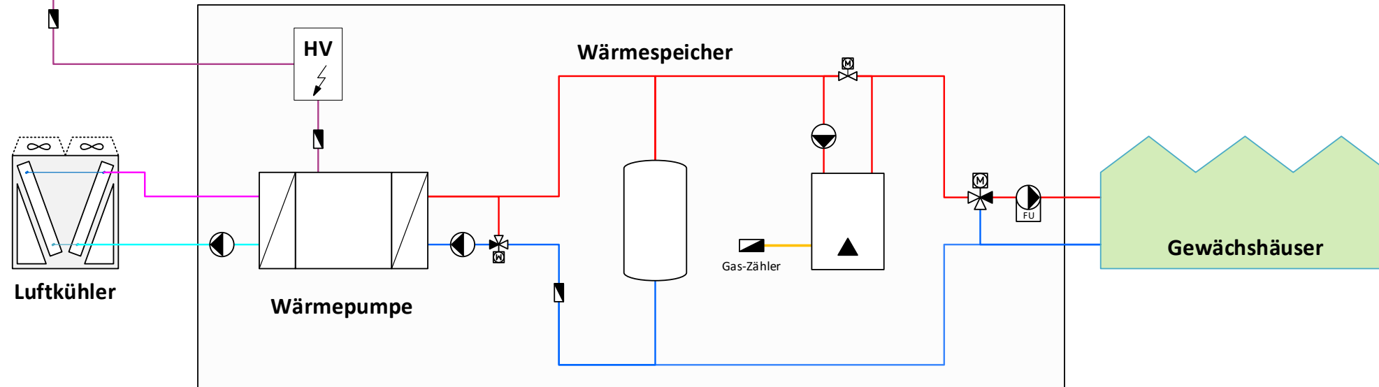
Heizzentrale
